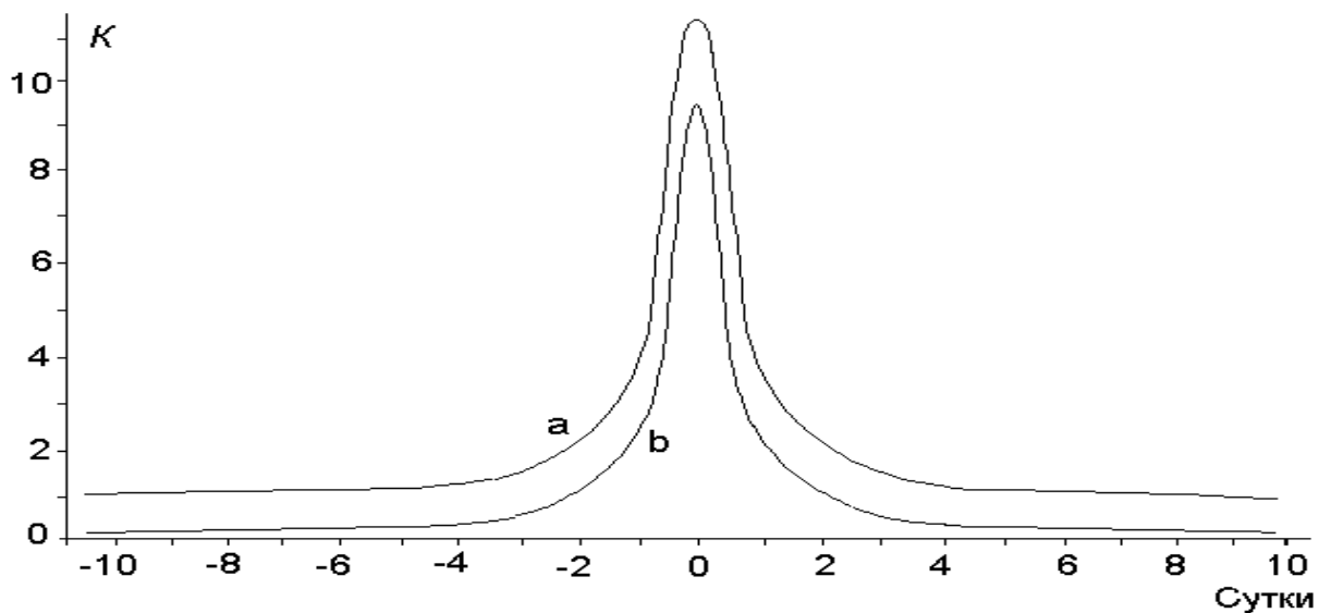
Рис. 5. Расчетное изменение плотности потока проходящих вблизи Солнца мононаправленных частиц, имеющих скорость 500 \text{ км/с} , при угловом сближении направления потока и направления на центр Солнца (минимальное расстояние – 12 угловых минут) [13]. По горизонтальной оси – время от момента наиболее тесного сближения; a – первичный "источник", b – возникающий и исчезающий "источник".
