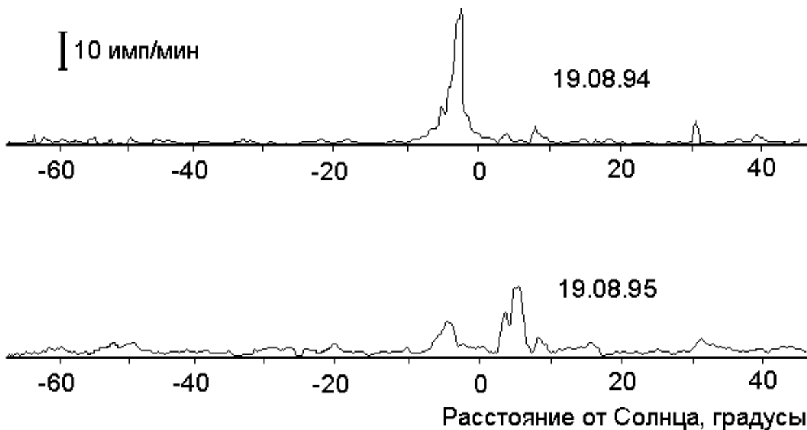
Рис. 6. Всплески сигнала во время сближения центра Солнца со звездой \nu Льва (минимальное расстояние 5 угловых минут). Телескоп: стальное параболическое зеркало с фокусным расстоянием 10 см, детектор – счетчик Гейгера диаметром 2 мм и длиной 6 мм [8].
