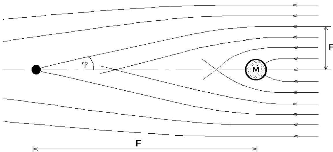
Рис. 3. Фокусировка неподвижным гравитирующим объектом. Проходящий со скоростью V на расстоянии от центра объекта p = (2GMF)^{1/2} / V поток агента "схлопывается" в точке наблюдения. Наблюдатель воспринимает приходящий поток как кольцо с угловым радиусом \varphi \approx p/F .
