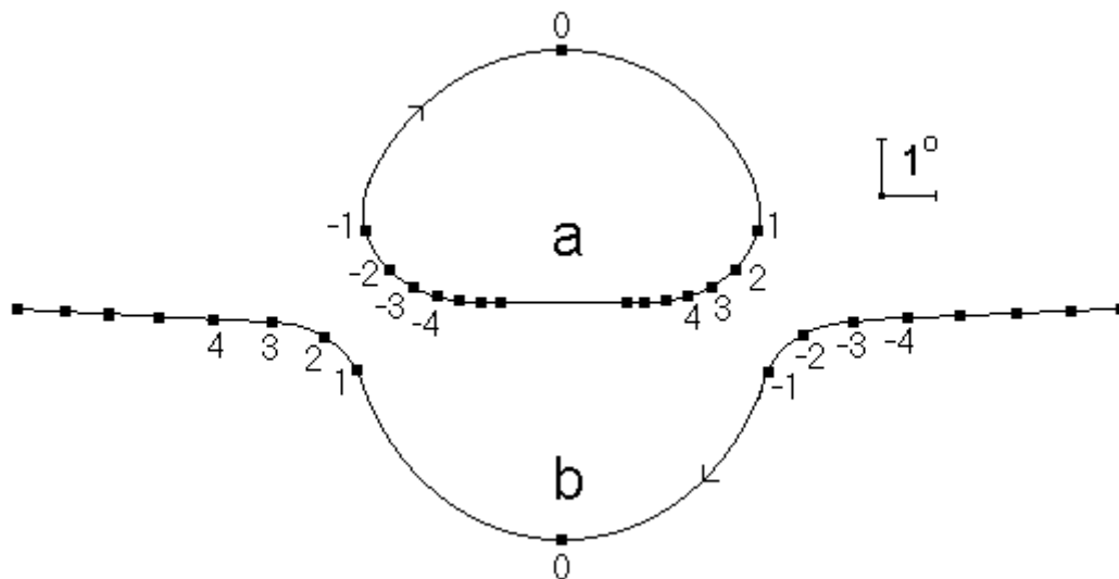
Рис. 4. Влияние Солнца на наблюдаемое положение относительно звезд источника потока частиц, имеющих скорость 500 \text{ км/с} , при тесном угловом сближении неотклоненного положения с центром Солнца (минимальное расстояние – 12 угловых минут) [13]. Цифрами обозначены наблюдаемые положения источника с интервалом в 1 сутки; нулю соответствует минимальное угловое расстояние между центром Солнца и неотклоненным направлением на источник; a – первичный "источник", b – возникающий и исчезающий "источник".
