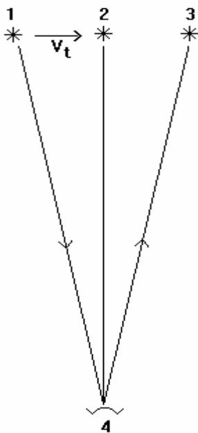
Рис. 2. "Прошрое" (1), "истинное" (2) и "будущее" (3) положения астрономического объекта. Порция света, излученная объектом, находящимся в положении (1), через много лет доходит до наблюдателя (4). За это время объект, двигающийся перпендикулярно направлению к наблюдателю со скоростью V_t , перемещается в положение (2). Если бы в момент регистрации порция света была бы излучена из места наблюдения, она встретилась бы с объектом в точке (3).
